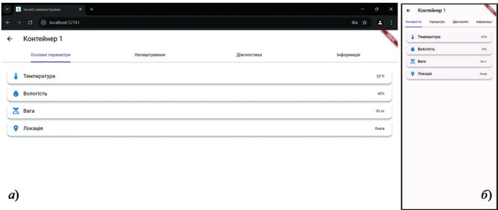
Рис. 3. Вкладка основних індикованих метрик
