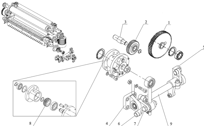
Частини механізму приводу розката друкарської секції № 2, що виходять з ладу
