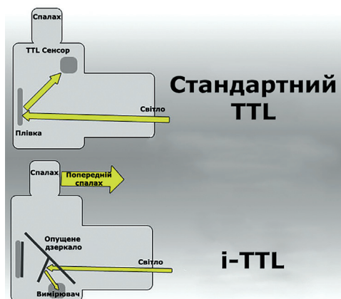
Принцип роботи систем вимірювання
