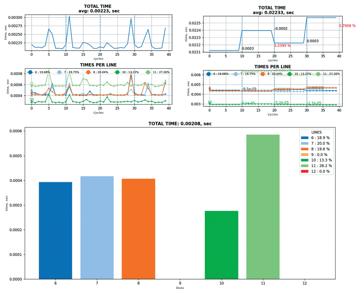
Графічний інтерфейс інструменту профілювання однопотоківих алгоритмів
