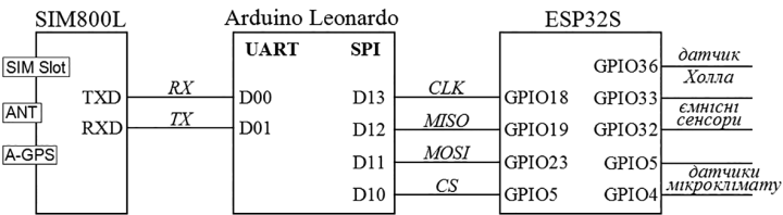
Апаратний інтерфейс підсистеми бездротового передавання індустриальних метрик
